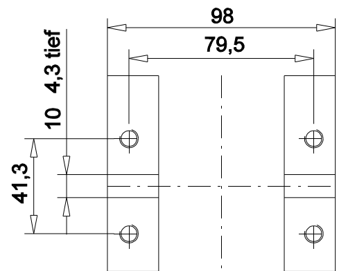
Maße - Getriebefuß
